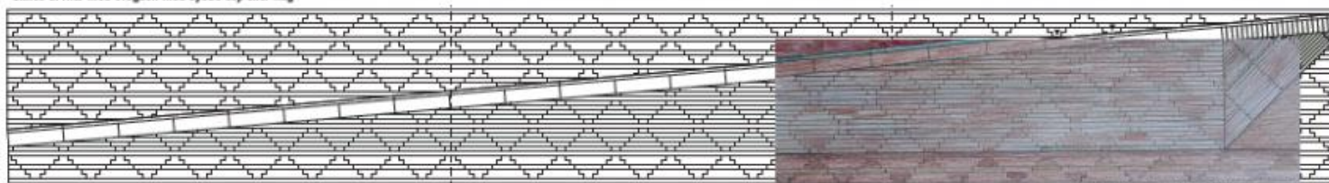
Mønsterplan af værkstøt med farveprøver på teglflade
